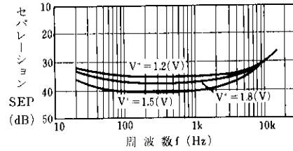
※セパレーション周波数特性例 ( V_{IN} = 150mV , T_a = 25^\circ\text{C} )
