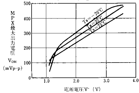
MPX最大出力電圧対電源電圧特性例 ( f = 1kHz , R_1 = 10k\Omega )
