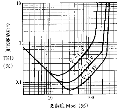
※全高調歪率対変調度特性例 ( f = 1kHz , T_a = 25^\circ\text{C} )
