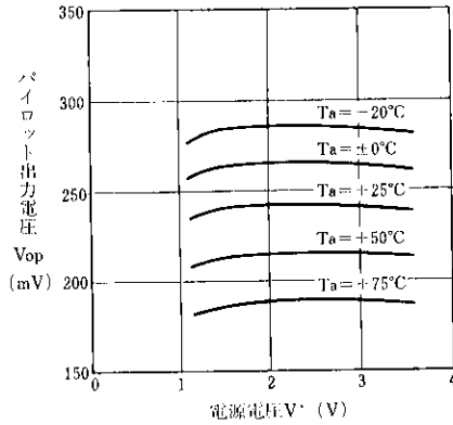
パイロット出力電圧対電源電圧特性例 ( R_1 = 150k\Omega )
