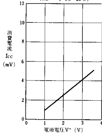
消費電流対電源電圧特性例 ( R_L = \infty, T_a = 25^\circ\text{C} )
