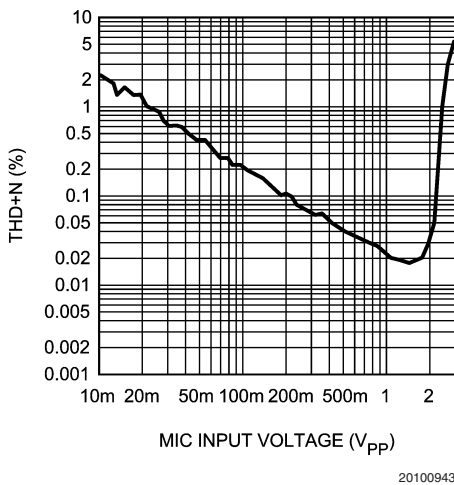
ADC THD+N vs MIC Input Voltage (MIC Gain = 6dB), AV DD = 5V
