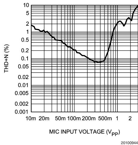
ADC THD+N vs MIC Input Voltage (MIC Gain = 6dB), AV DD = 3V
