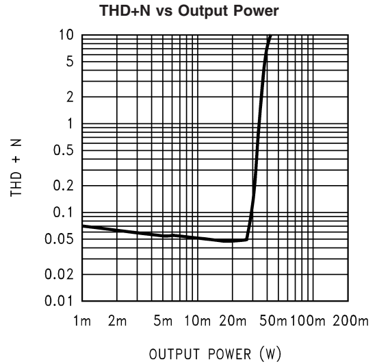
20079725 V_{DD} = 3V ; EP; f = 1kHz ; R_L = 32\Omega ; Mode 1; 0dB Gain
